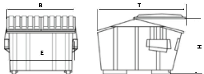
Front- und Seitenansicht des Frontladerbehälters
